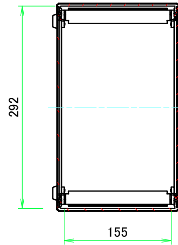
A-A ( 1 :5.5 )
